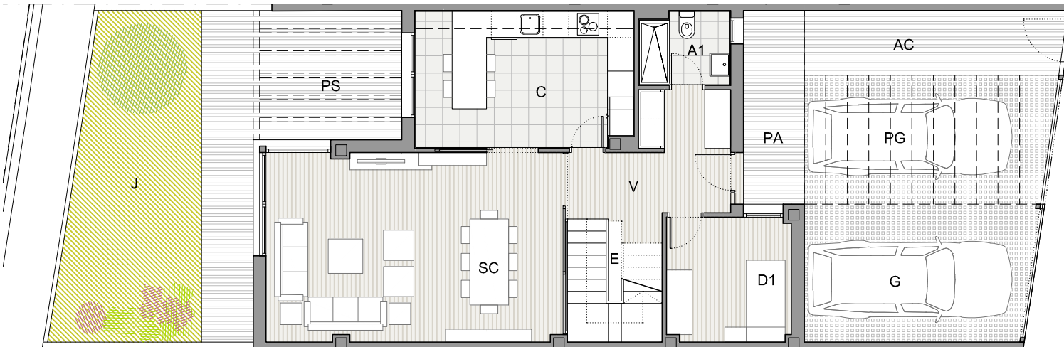
PLANTA BAJA E 1/125
