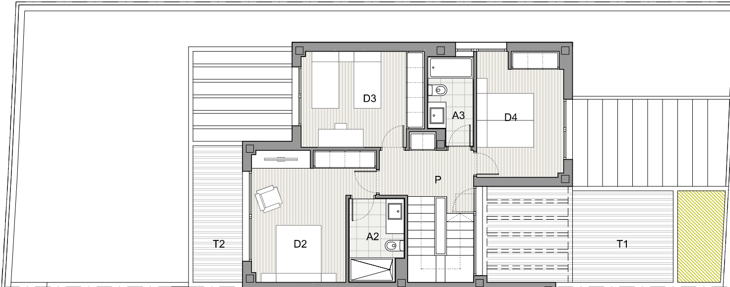
PLANTA PRIMERA E 1/125
