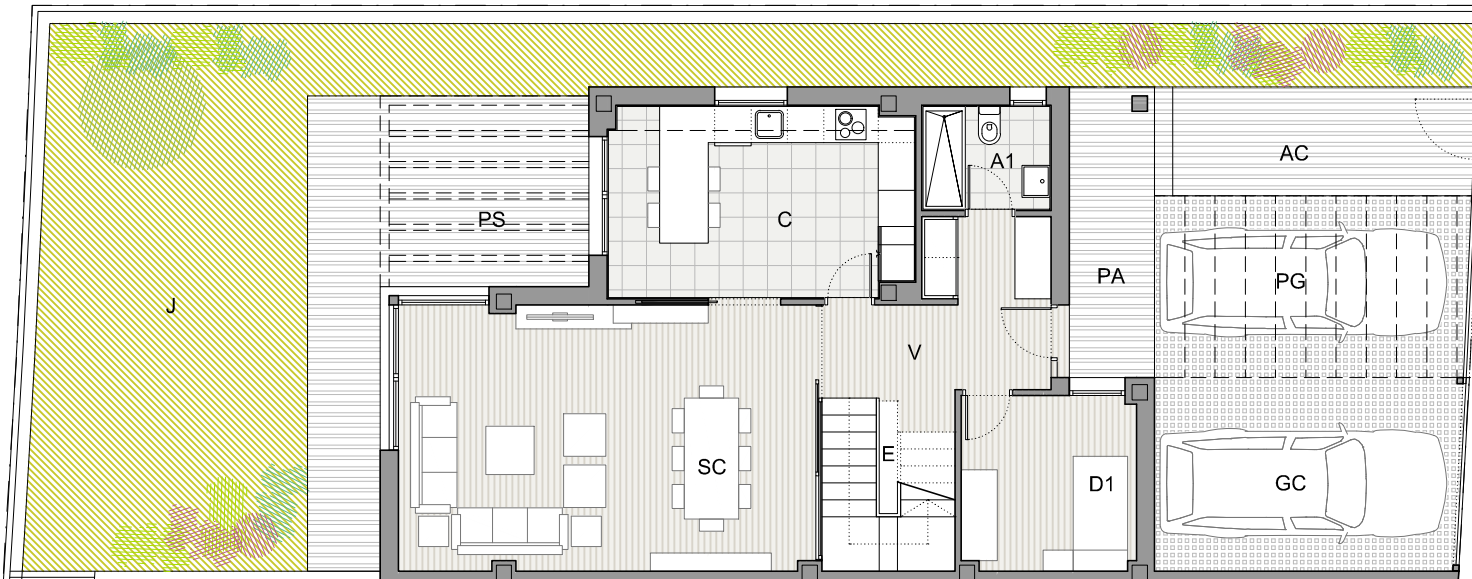
PLANTA BAJA E 1/125
