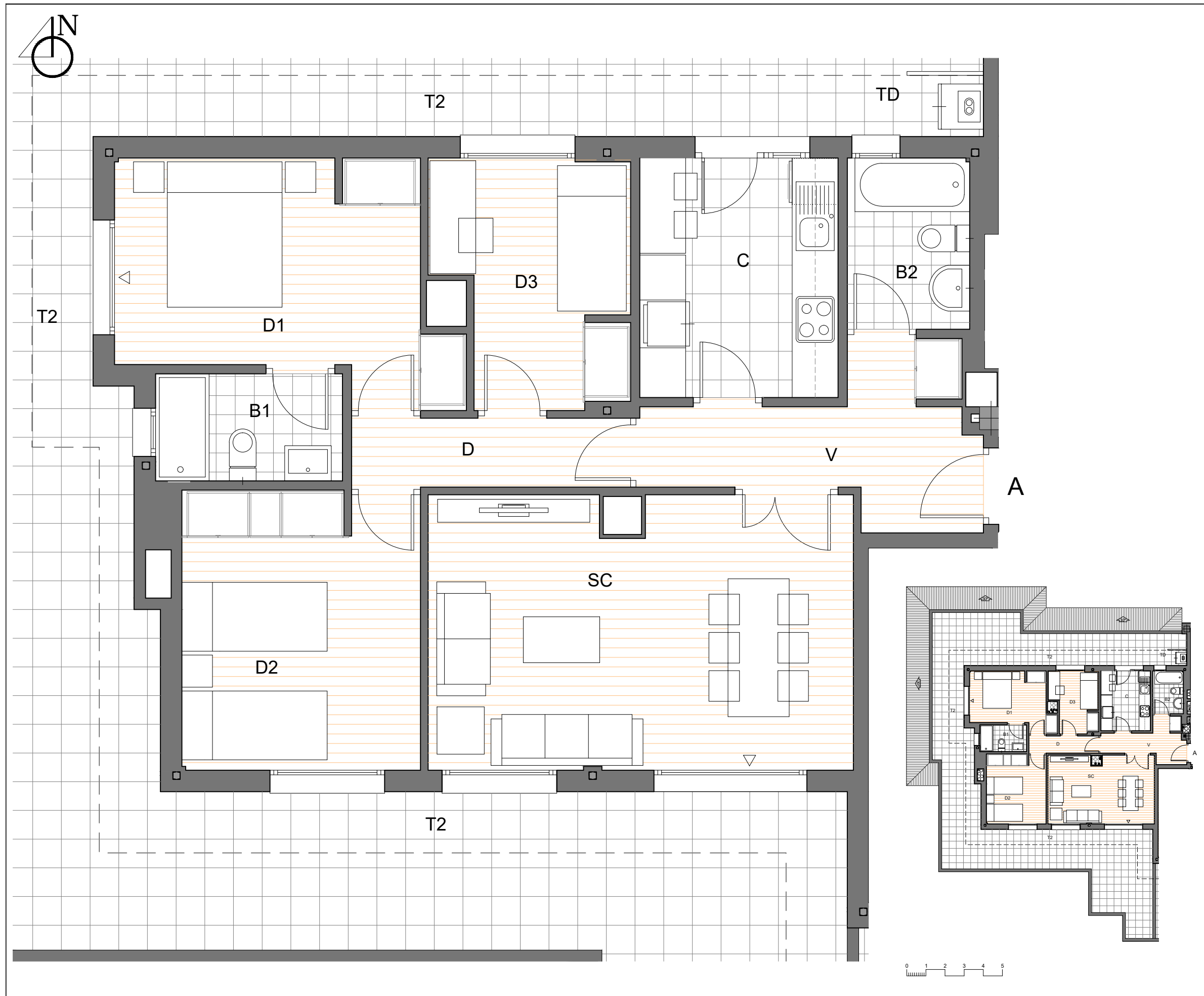
PLANTA ÁTICO
