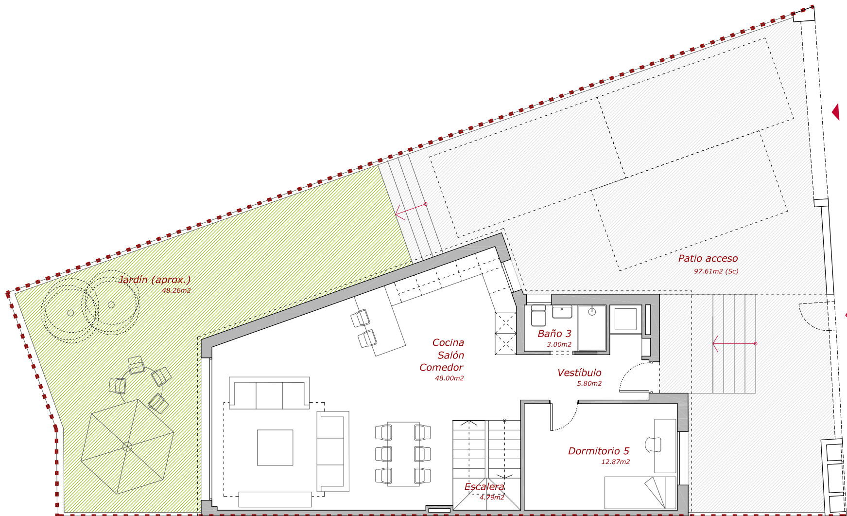
PLANTA BAJA
