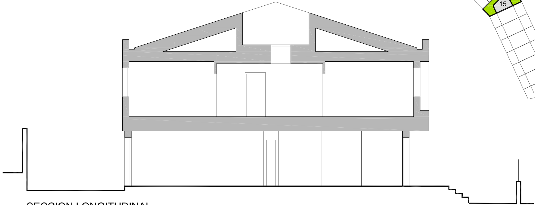
SECCION LONGITUDINAL
